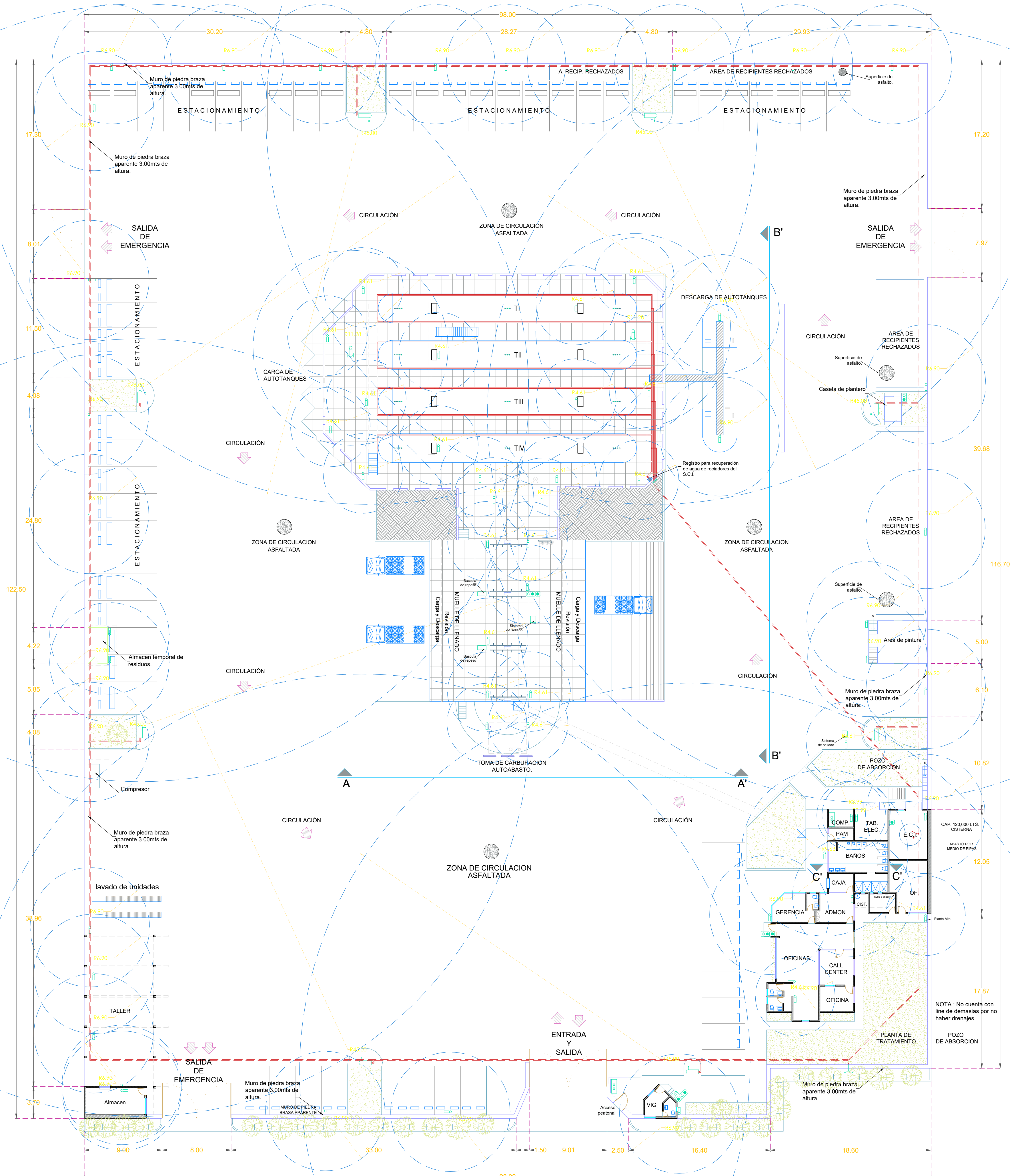
Planta S.C.I. ESC 1:250
