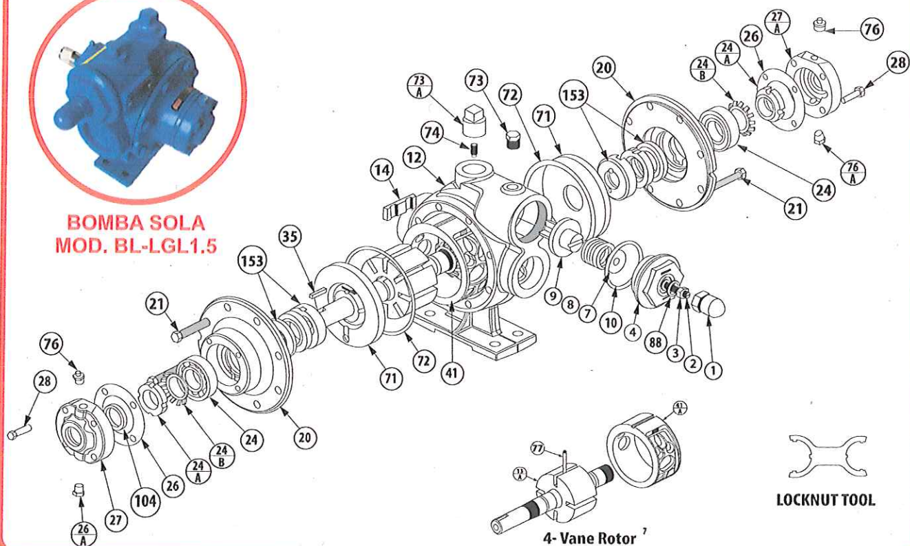
4- Vane Rotor
