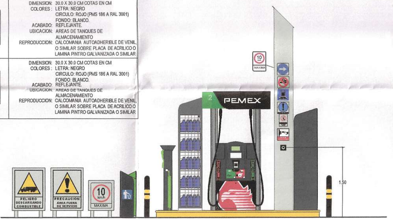
DETALLE ESCALA 1:50
