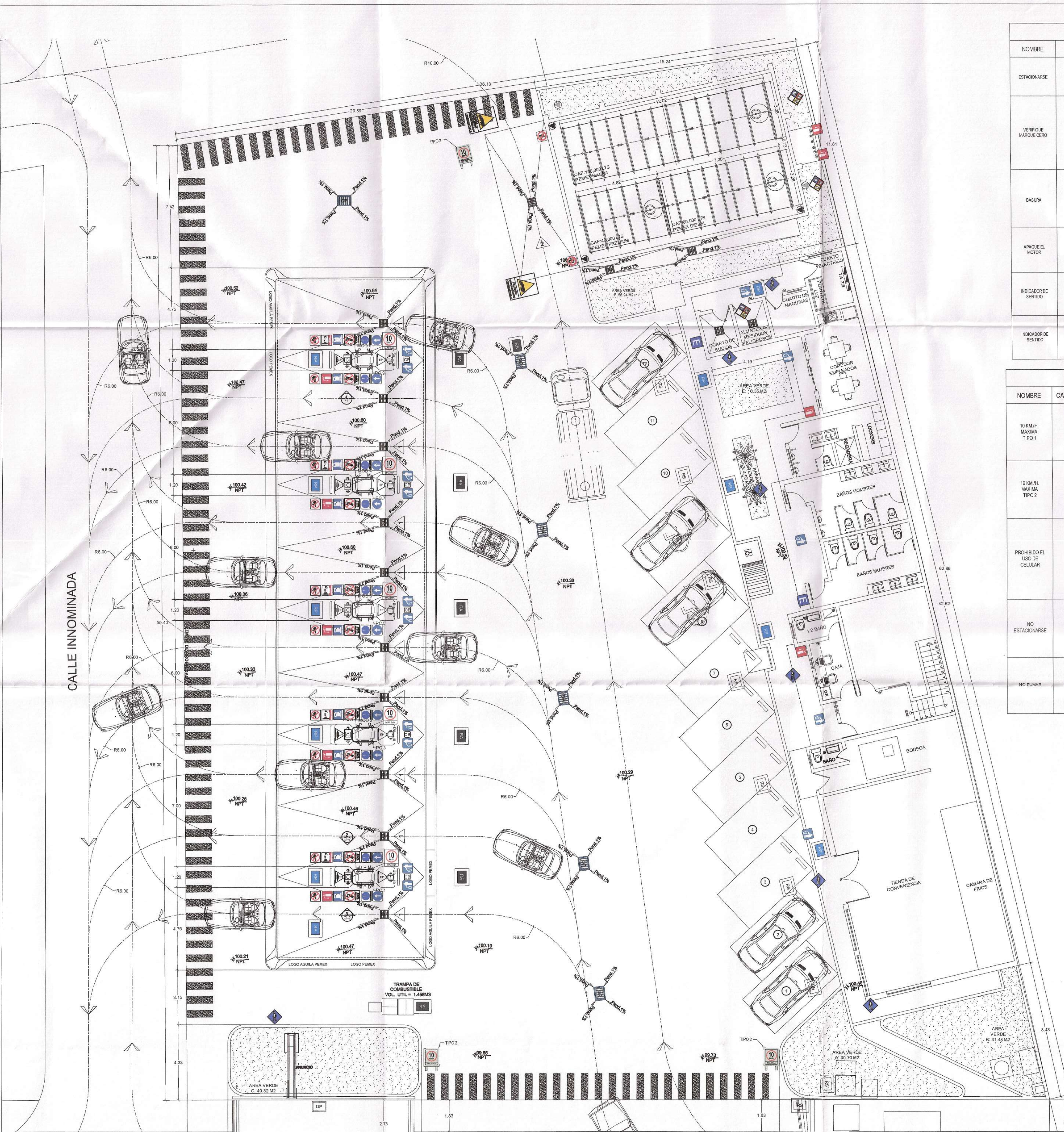
DISTRIBUCION GENERAL ESCALA 1:125
