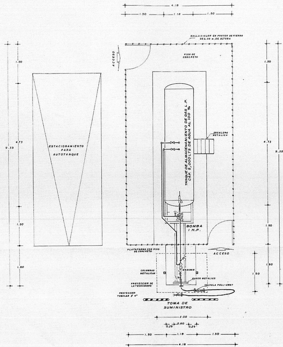
DIAGRAMA EN PLANTA DE LA INSTALACION DE TRASIEGO ESC. 1:40
