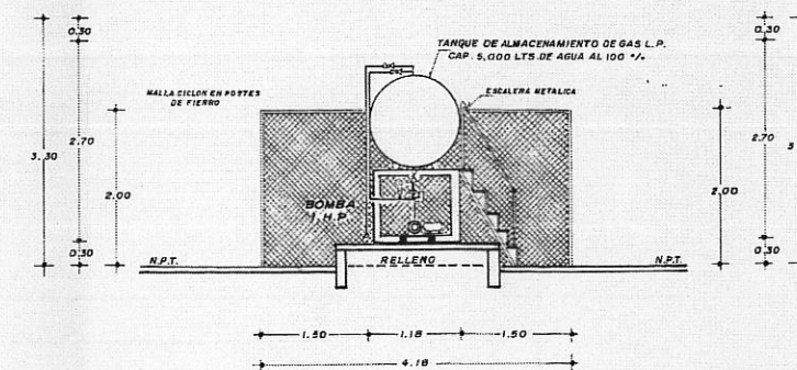
CORTE ELEVACION TRANSVERSAL DE ZONA DE ALMACENAMIENTO ESC. 1:50
