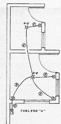
DETALLE No. 2 OFICINA Y BAÑO (S/E)
