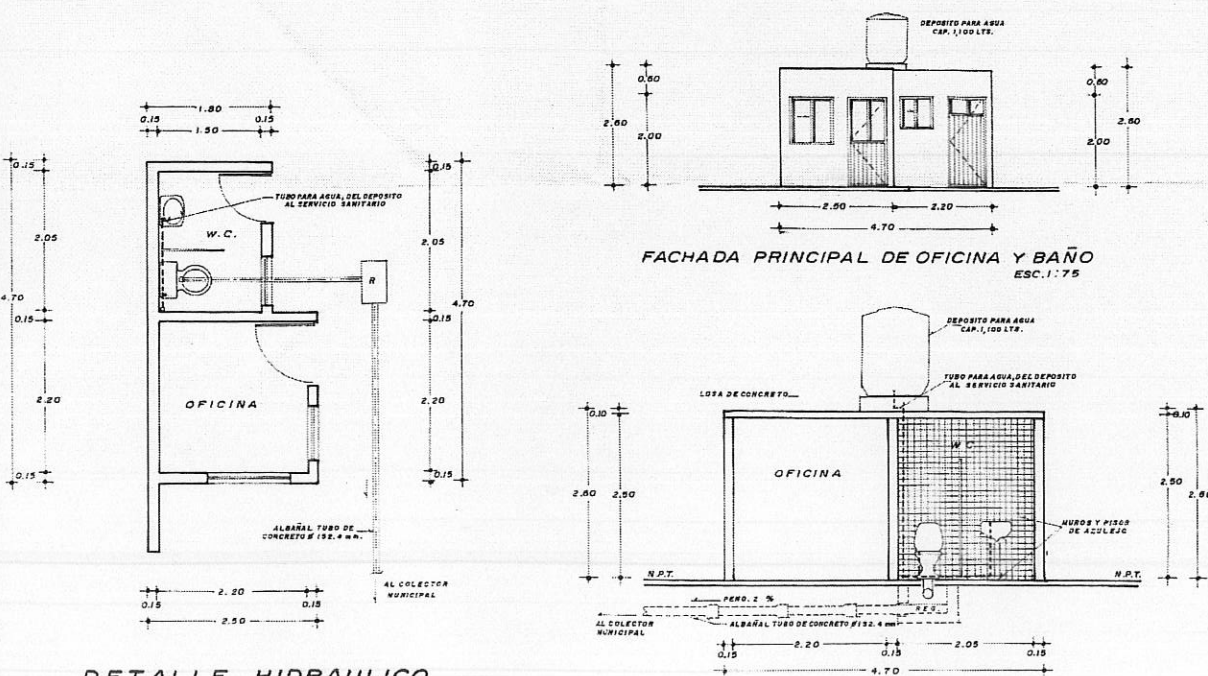
DETALLE HIDRAULICO
