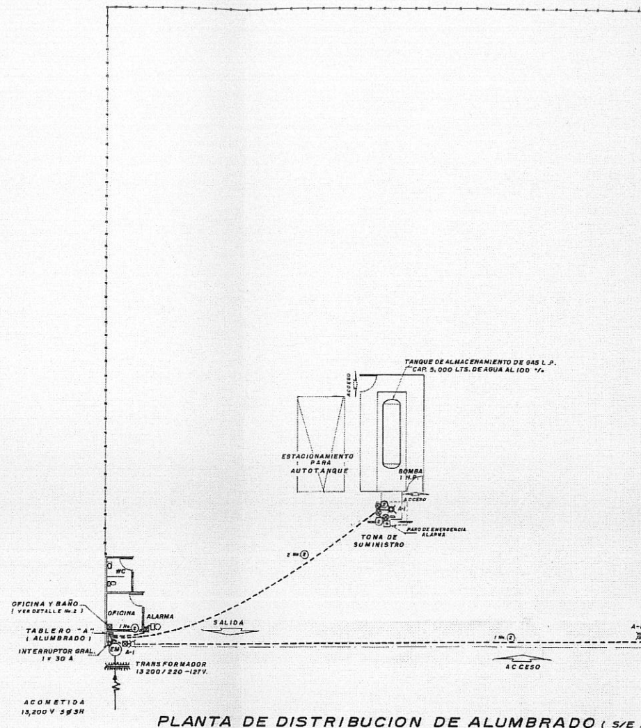
PLANTA DE DISTRIBUCION DE ALUMBRADO (S/E)
