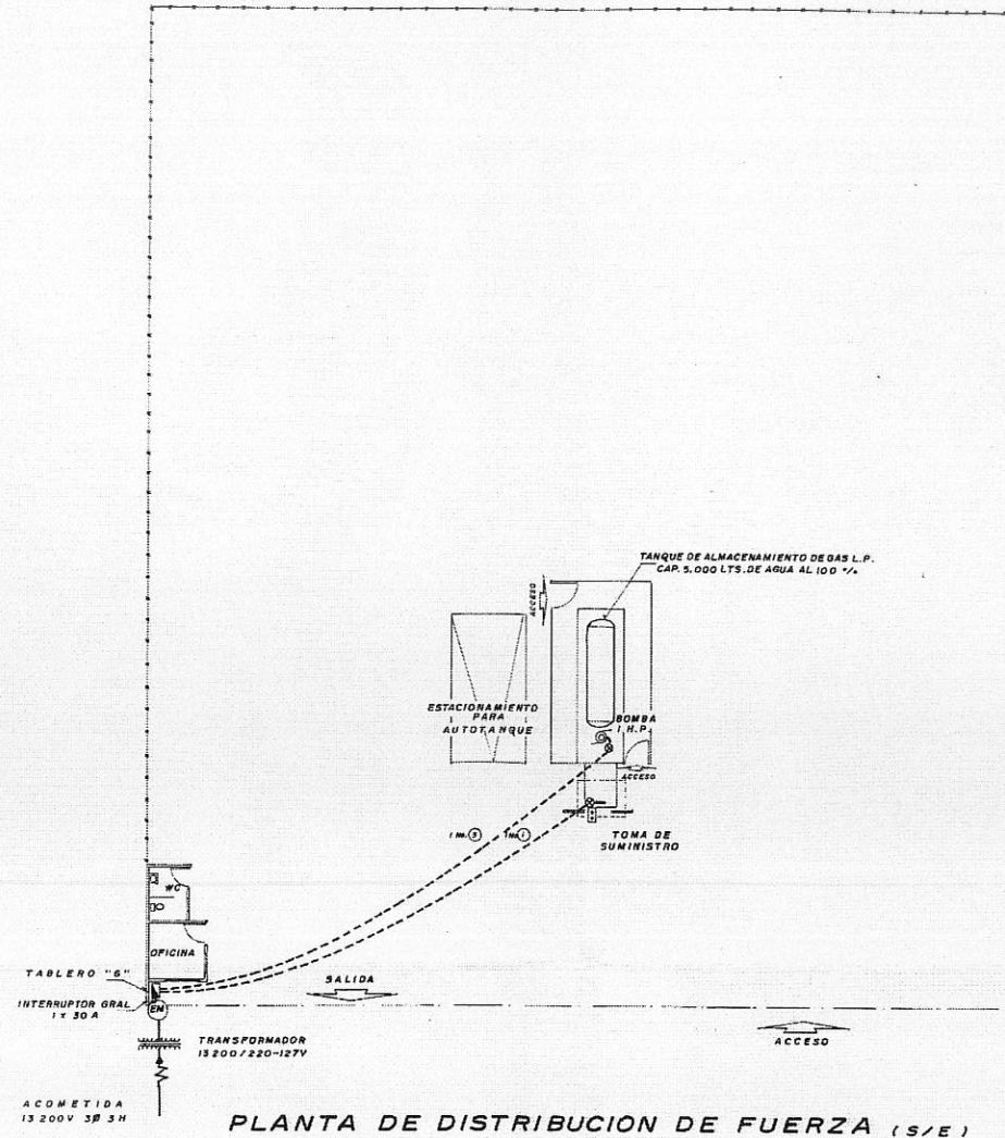
PLANTA DE DISTRIBUCION DE FUERZA (S/E)
