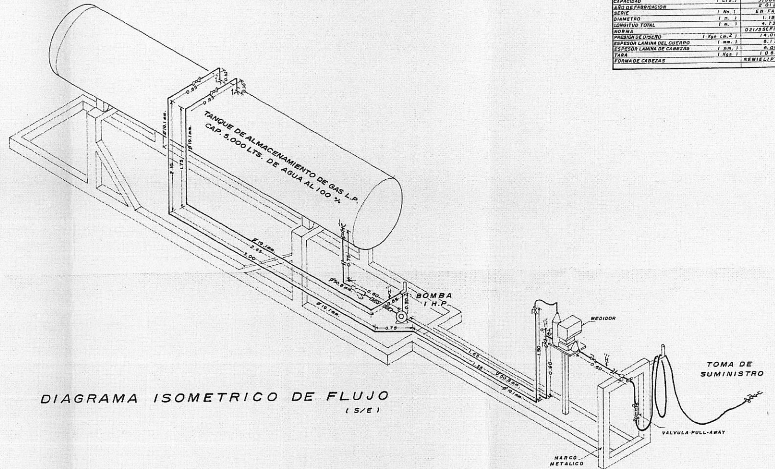
TANQUE DE ALMACENAMIENTO DE GAS L.P. ESC. 1:50
