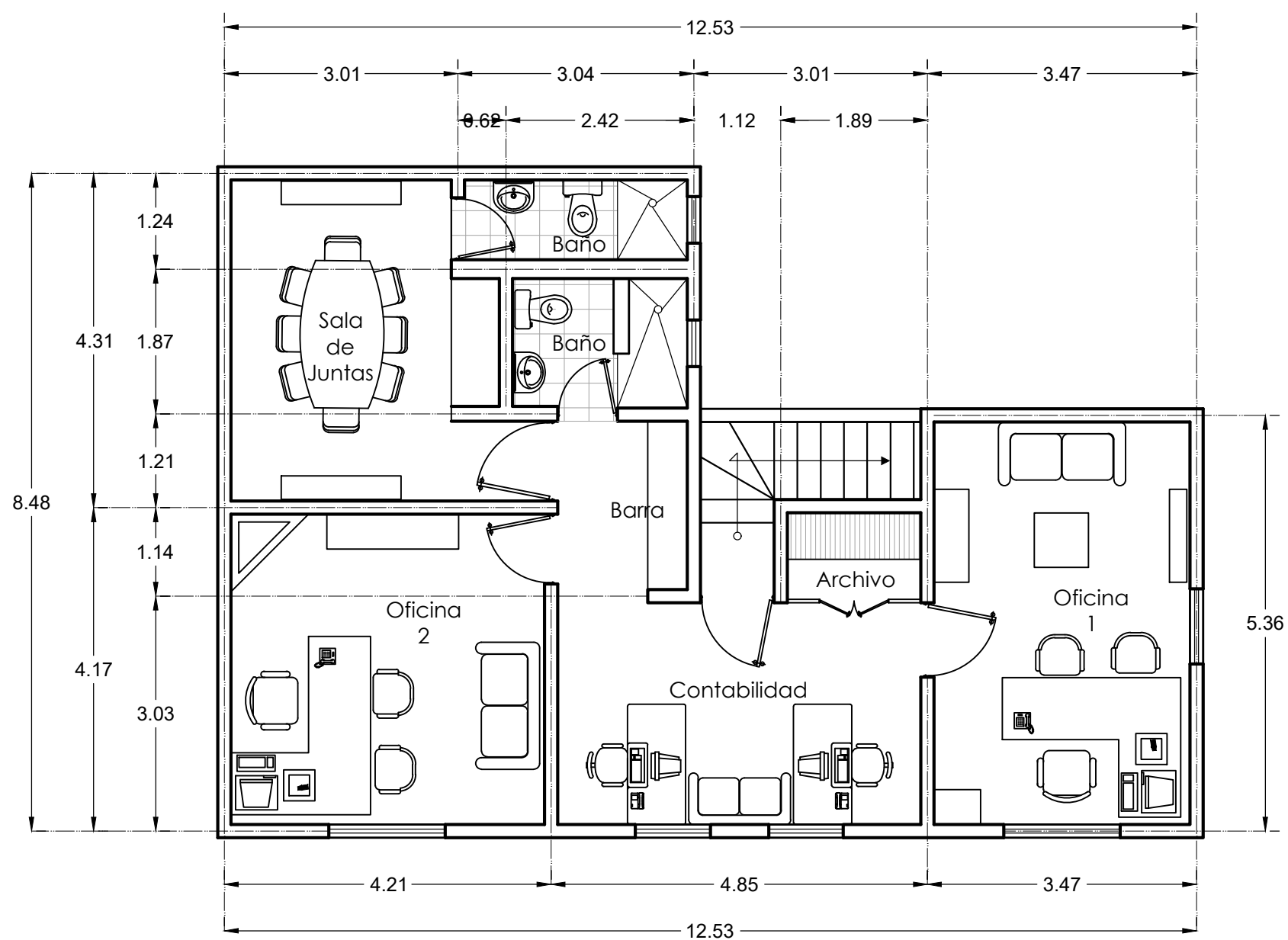
1 PLANTA ARQUITECTONCIA ALTA Escala: 1:75
