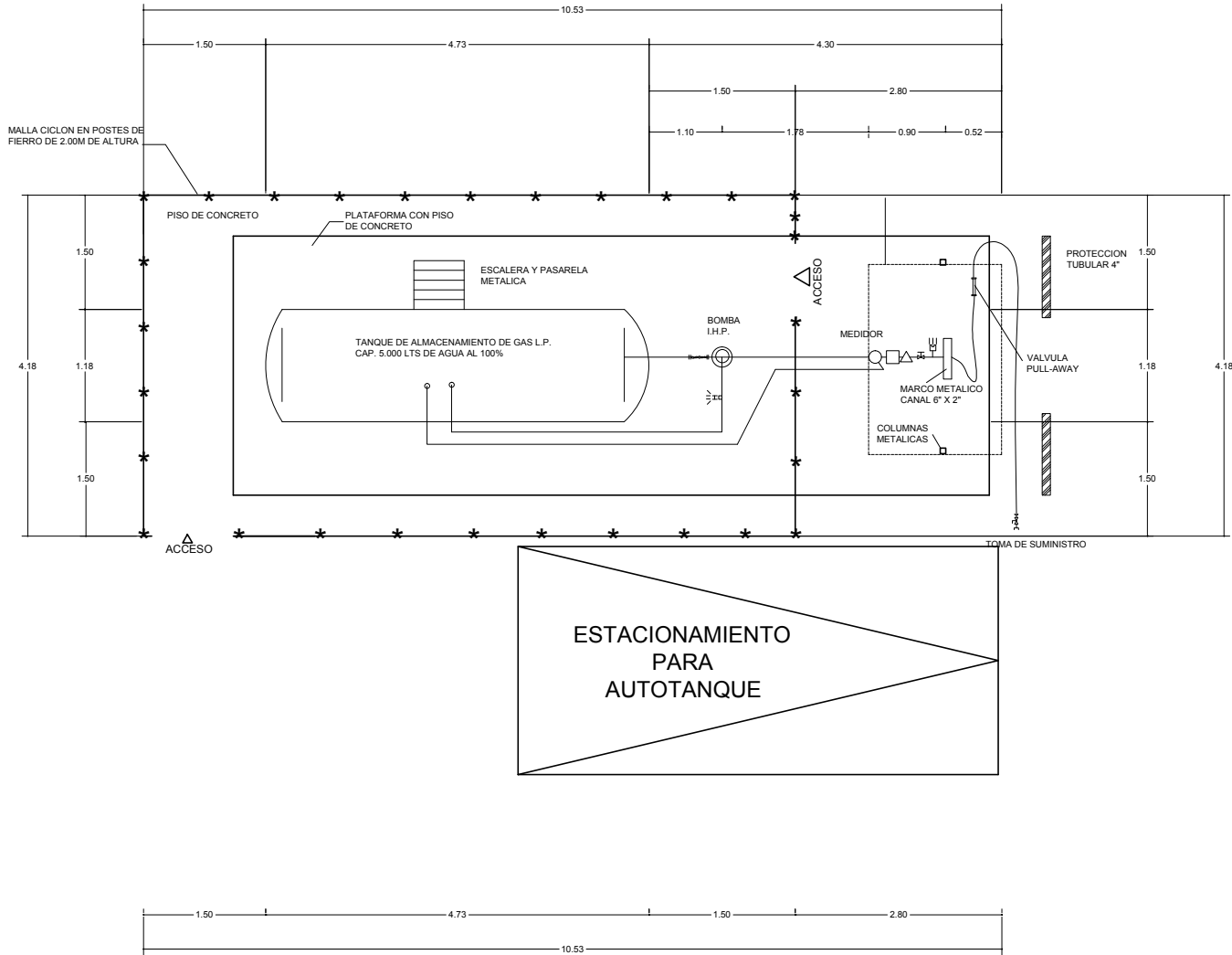
DIAGRAMA EN PLANTA DE LA INSTALACION DE TRASIEGO S/E
