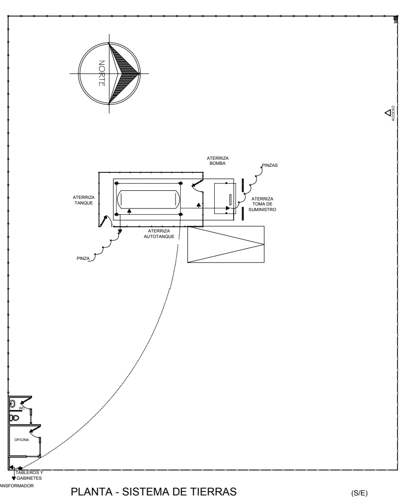
PLANTA - SISTEMA DE TIERRAS (S/E)
