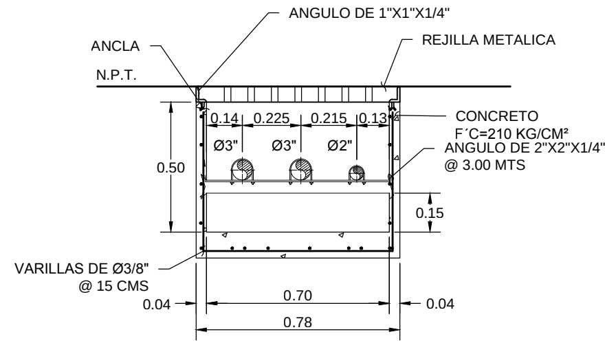
DETALLE 1 - DUCTO DE CONCRETO ISLETA DE TOMA DE CARGA A AUTO-TANQUES ESC. 1:20
