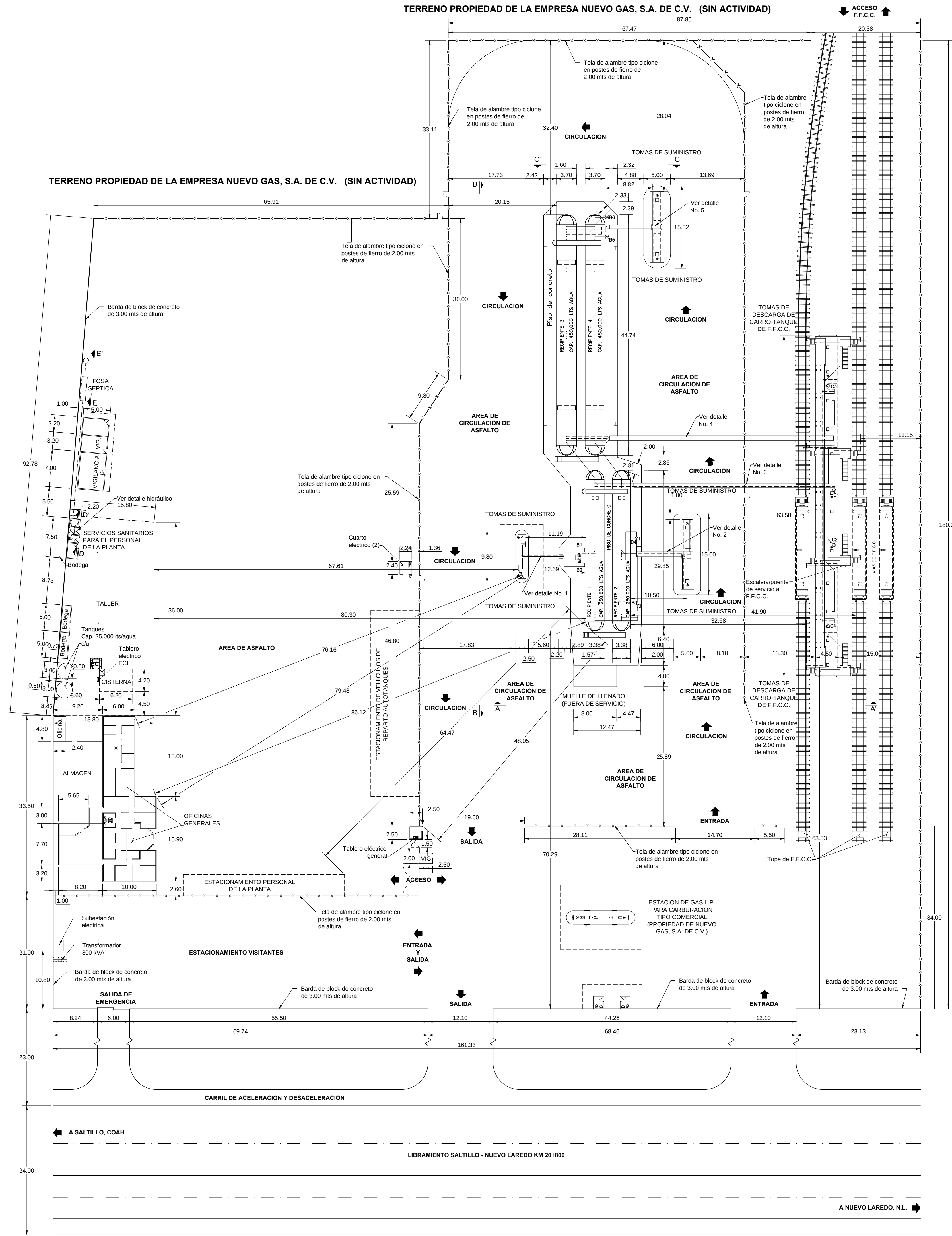
PLANO DE DISTRIBUCION DE EQUIPO ESC. 1:400
