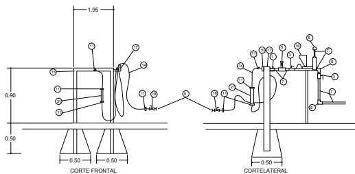
ANCLAJE DE LA TOMA (S/E)
