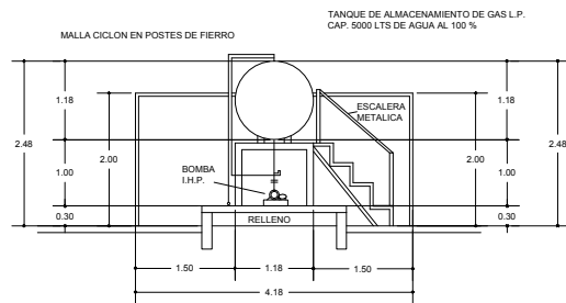
CORTE ELEVACION TRANSVERSAL DE ZONA DE ALMACENAMIENTO
