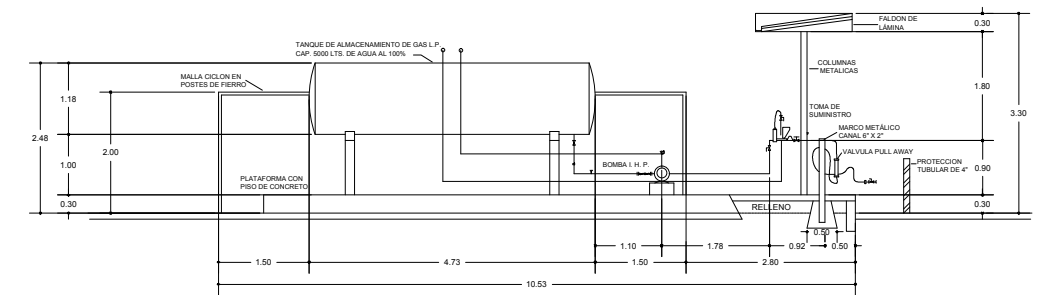
CORTE ELEVACION LONGITUDINAL DE ZONA DE ALMACENAMIENTO Y LATERAL DE TOMA DE SUMINISTRO
