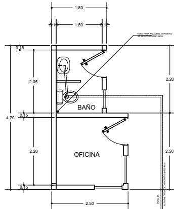
DETALLE HIDRAULICO
