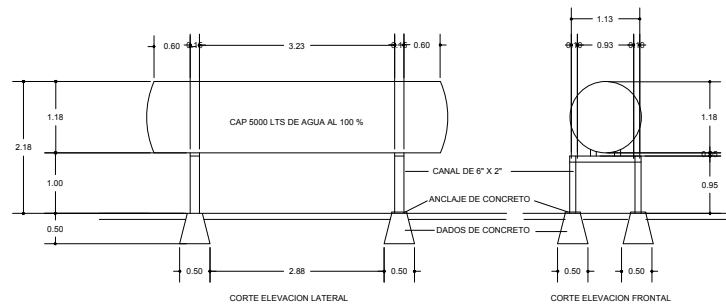
BASES DE SUSTENTACION DEL TANQUE PARA GAS L.P.
