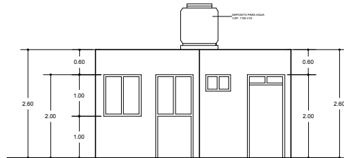
FACHADA PRINCIPAL DE OFICINA Y BAÑO
