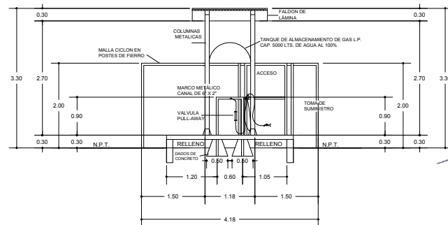
CORTE ELEVACION FRONTAL DE TOMA DE SUMINISTRO
