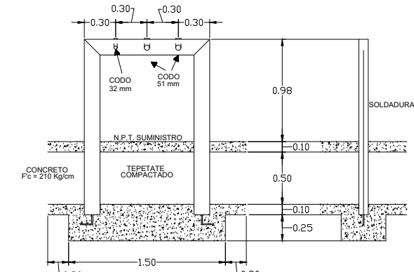
DETALLE DE SOPORTE METÁLICO PARA TOMAS DE SUMINISTRO 1
