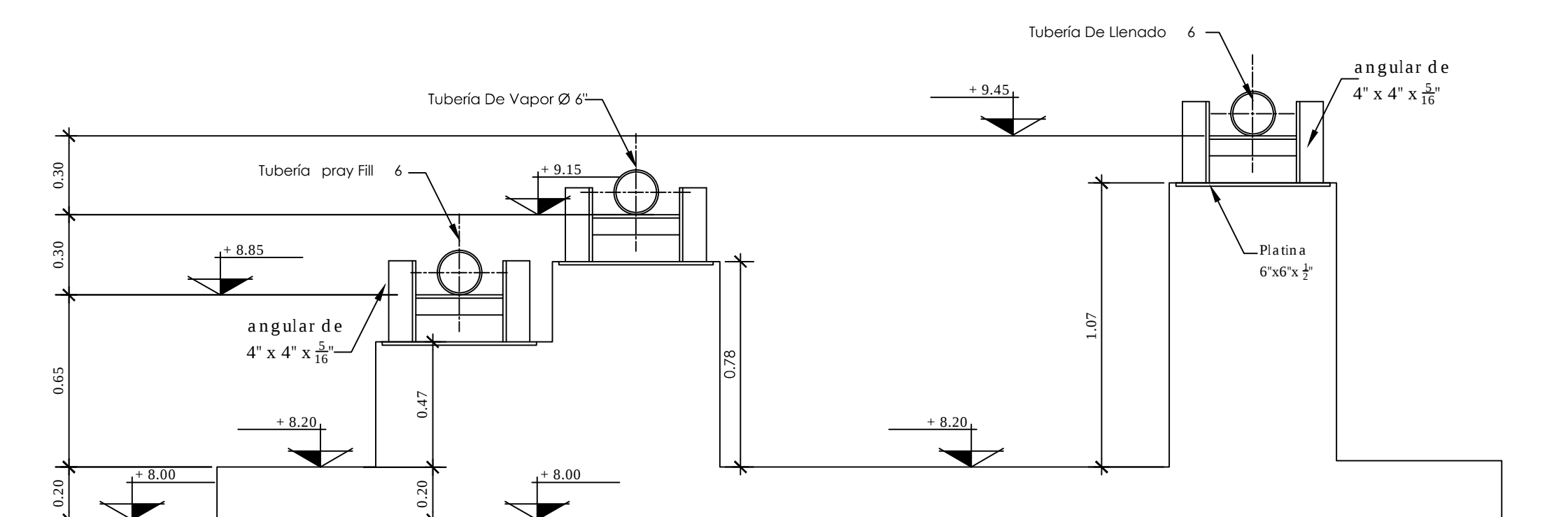
3 ALZADO TIPO SOPORTES A DE TUBERIA ESCALA 1:20
