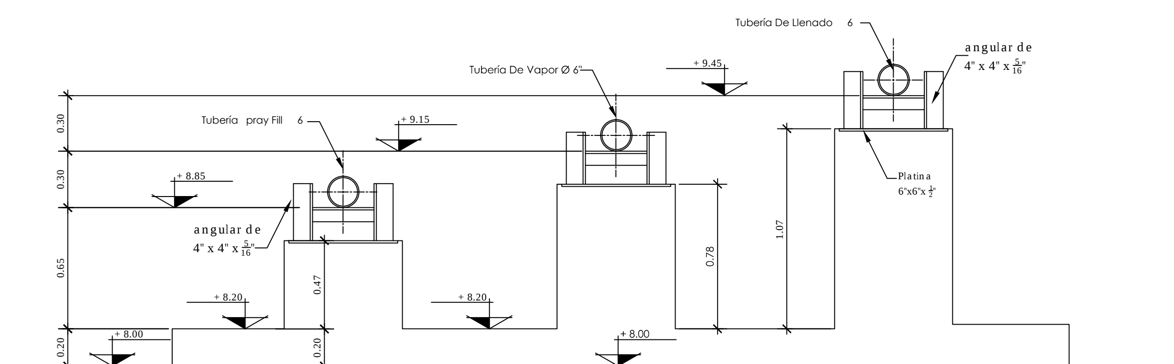
6 ALZADO TIPO SOPORTES B DE TUBERIA ESCALA 1:20
