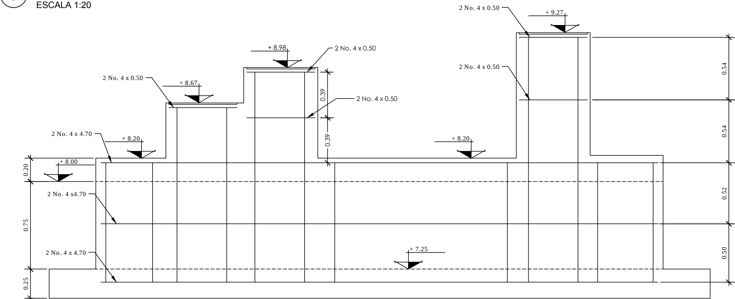
2 ELEVACION TIPO SOPORTES A DE TUBERIA ARMADO ESCALA 1:20
