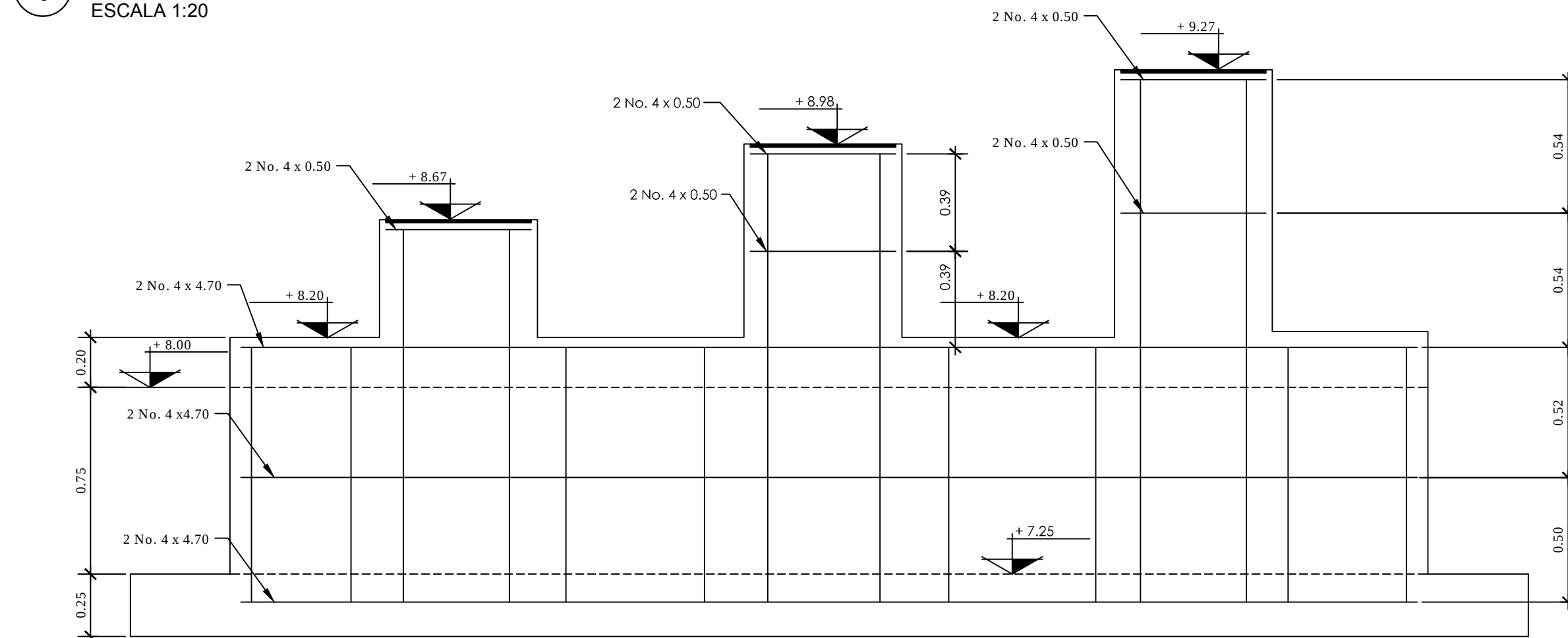
5 ELEVACION TIPO SOPORTES B DE TUBERIA ARMADO ESCALA 1:20
