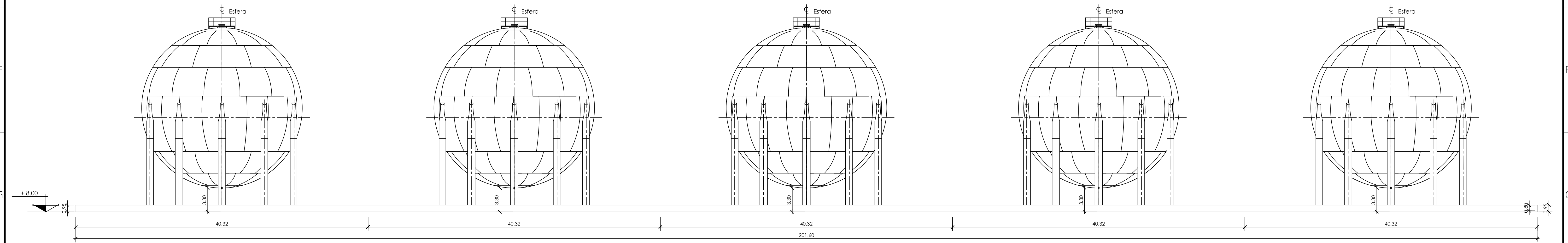
2 ELEVACION ZONA DE ALMACENAMIENTO GRUPO DE 5 ESFERAS ESCALA 1:250
