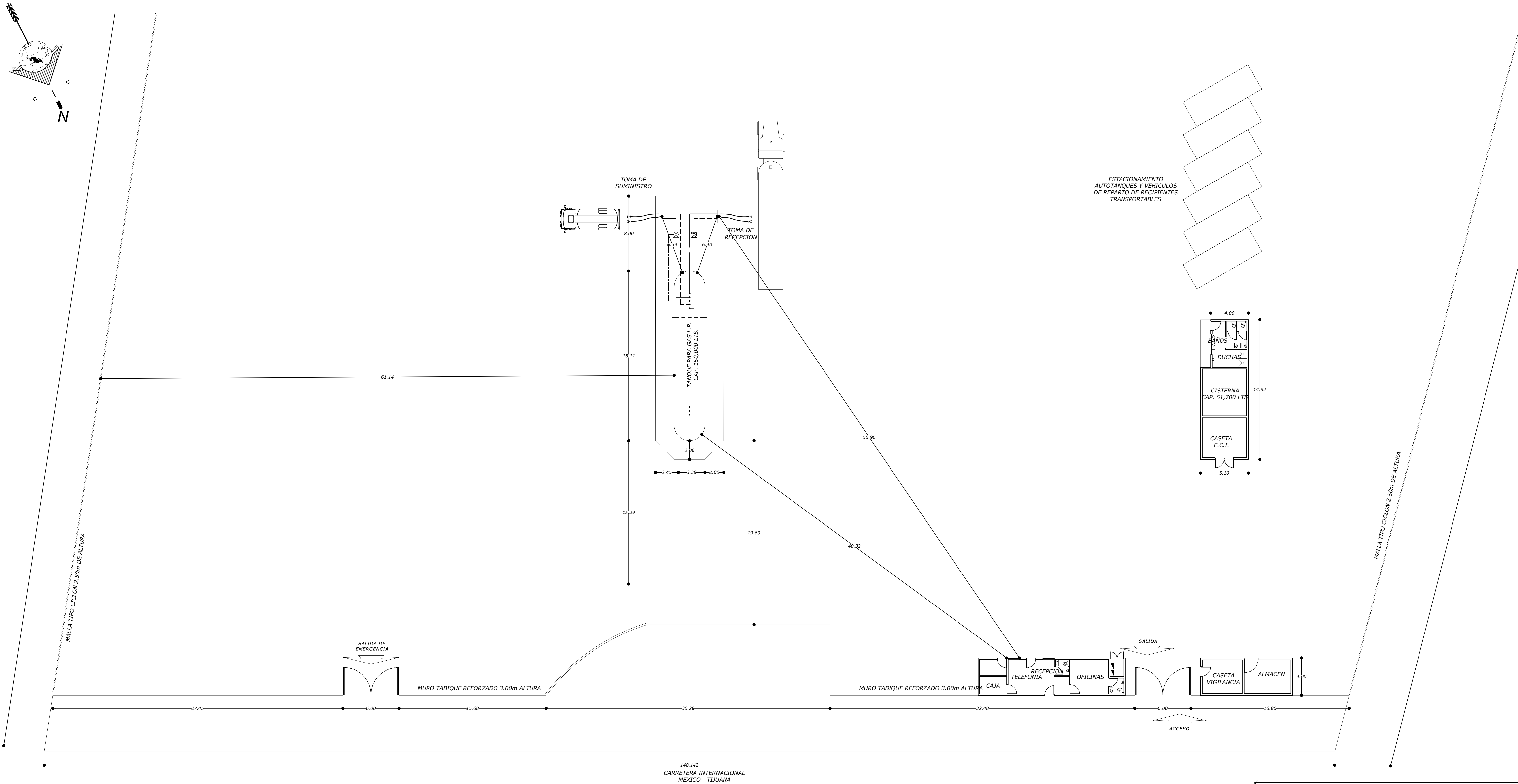
PLANTA DE DISTRIBUCION DE EQUIPO ESC. 1:200
