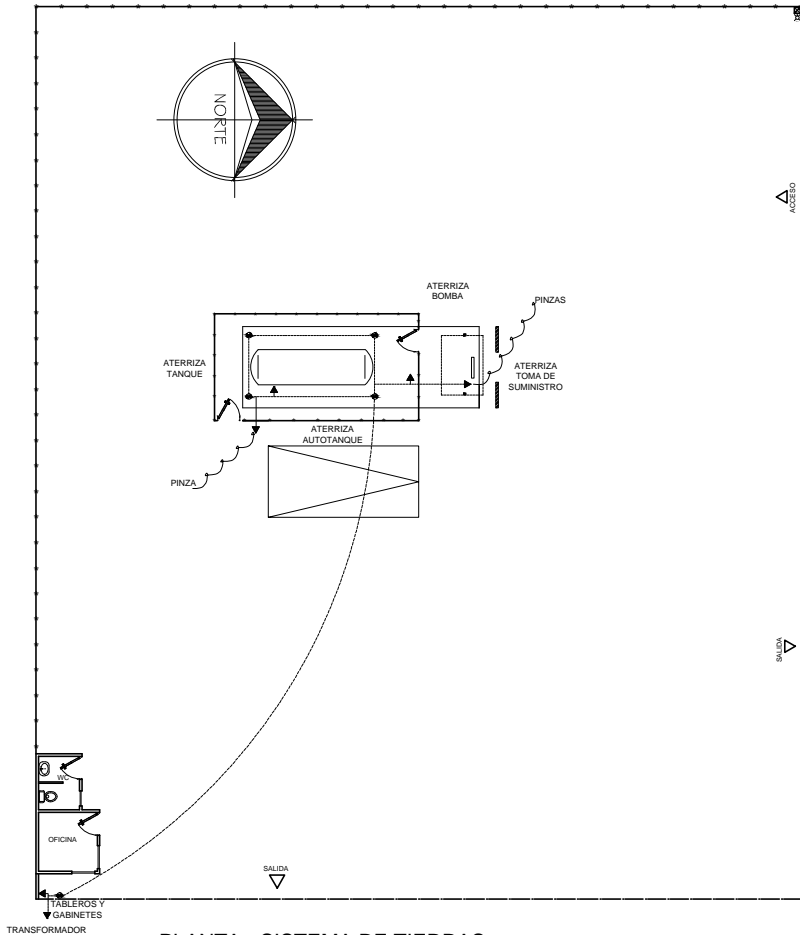
PLANTA - SISTEMA DE TIERRAS
